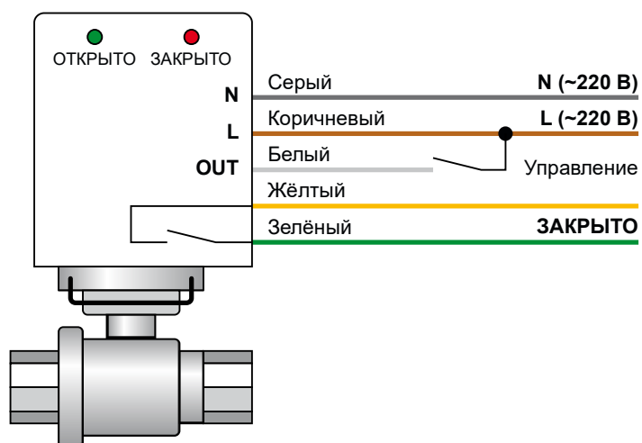
Рис. 3. Схема подключения и управления электроприводом Professional 220 BS FB.
